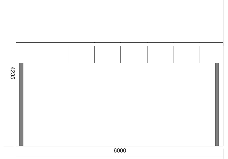
Right Elevation
